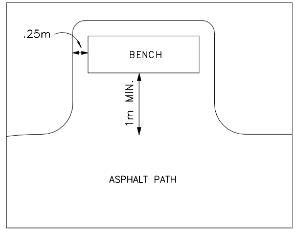
LAYOUT N.T.S.
