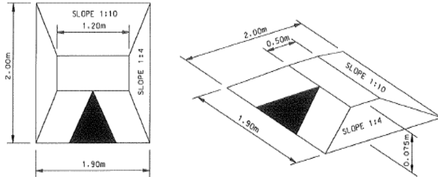
DIMENSIONS
