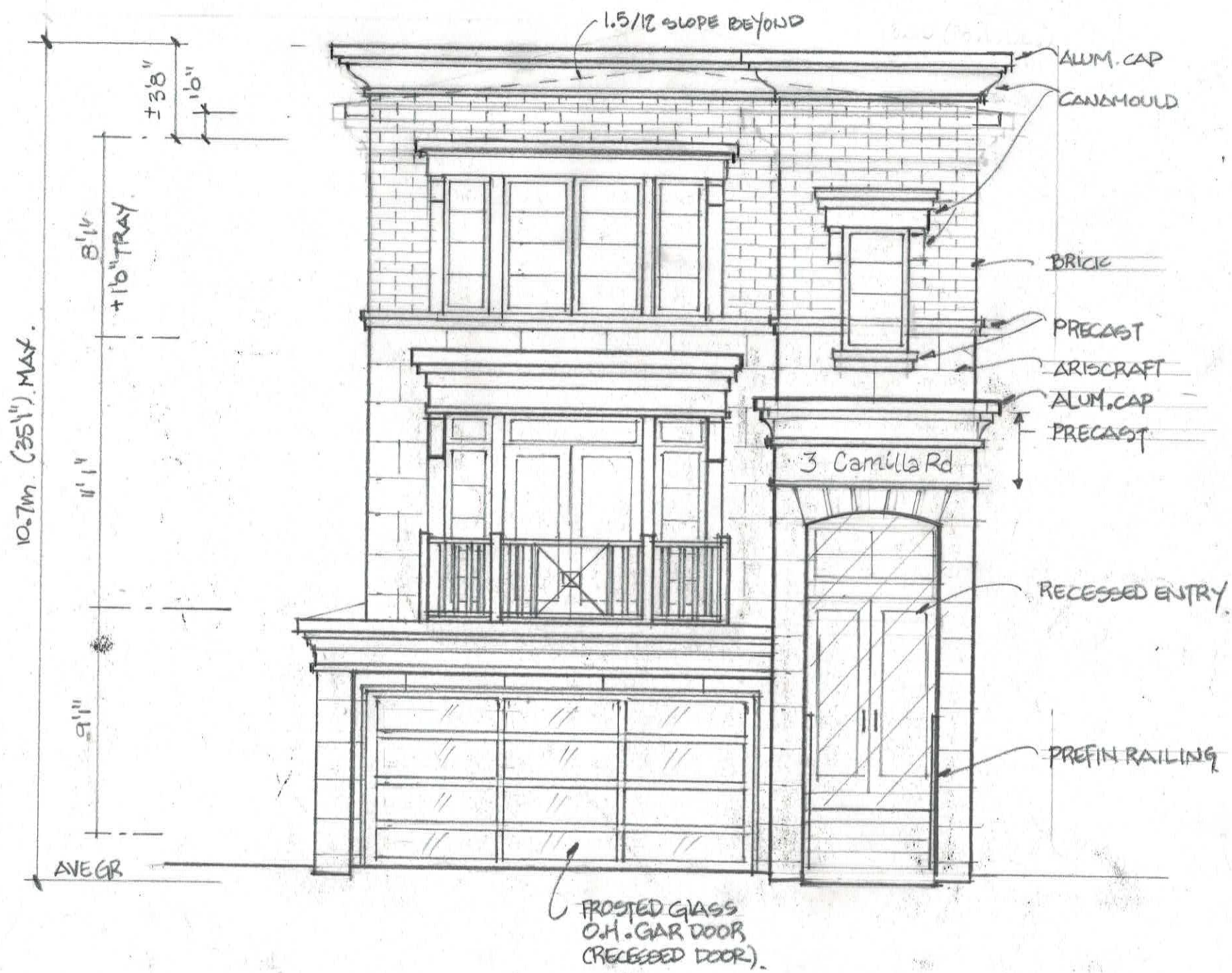
ELEVATION A.
