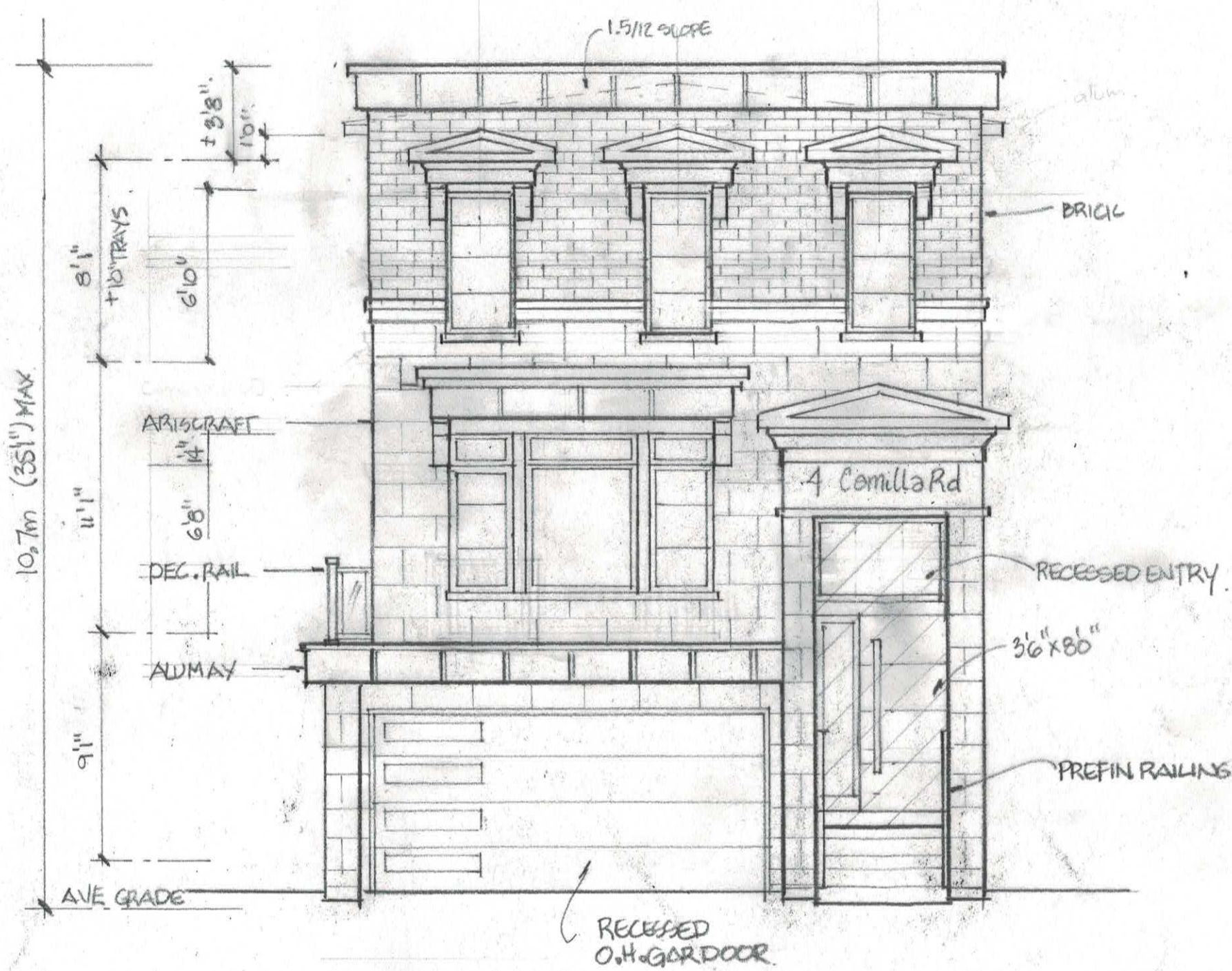
ELEVATION B.
