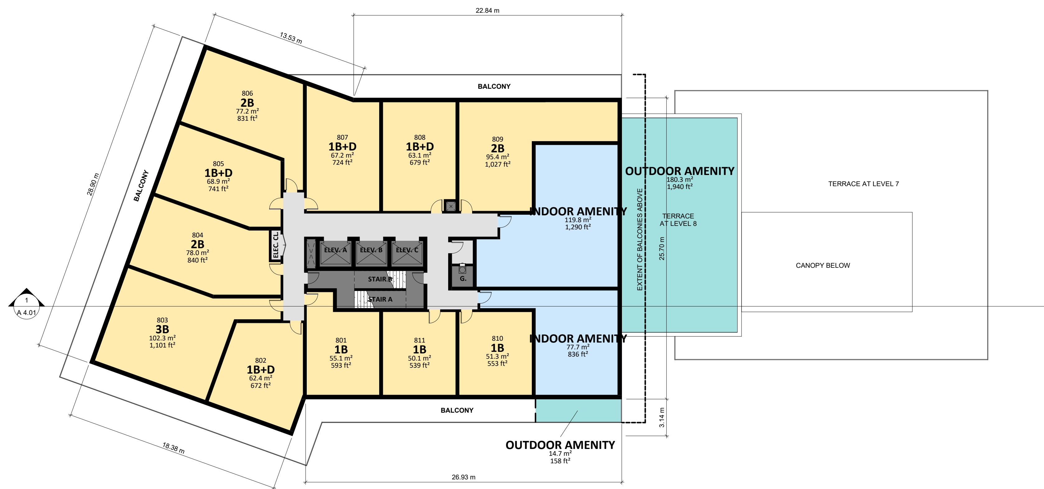
② LEVEL 8 1 : 200
