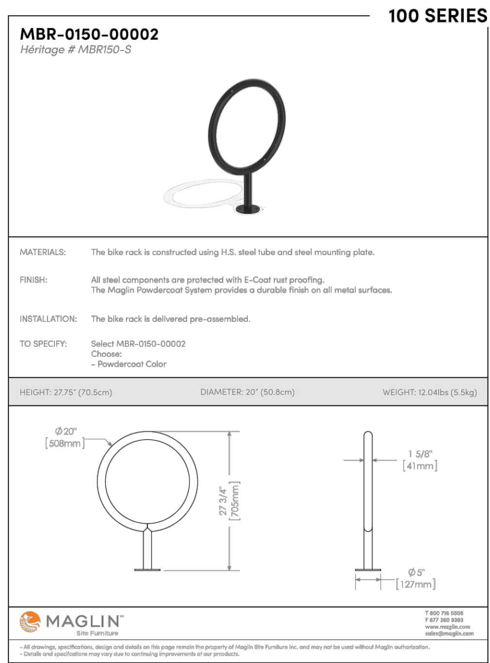
D5 BICYCLE PARKING SCALE: N.T.S.
