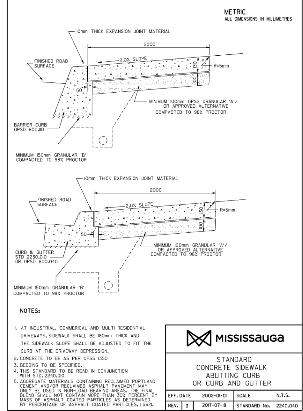
D6 STANDARD CONCRETE SIDEWALK SCALE: N.T.S.
