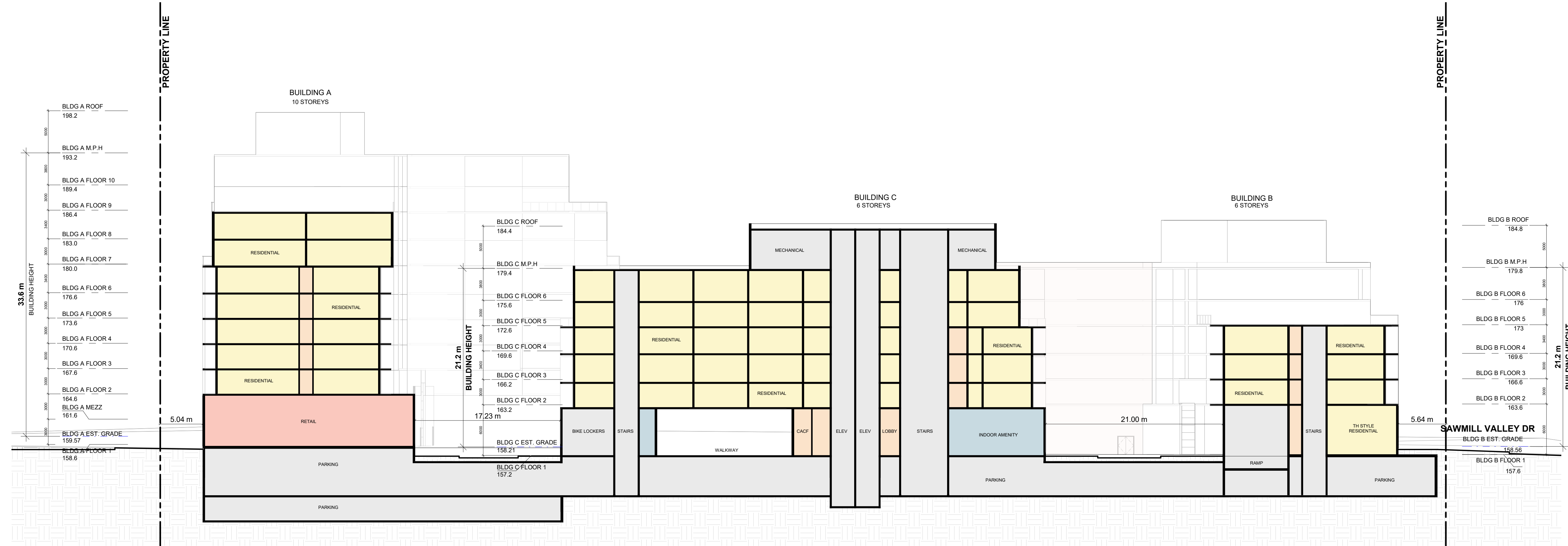
1 W-E SITE SECTION SPA402 1 : 250
