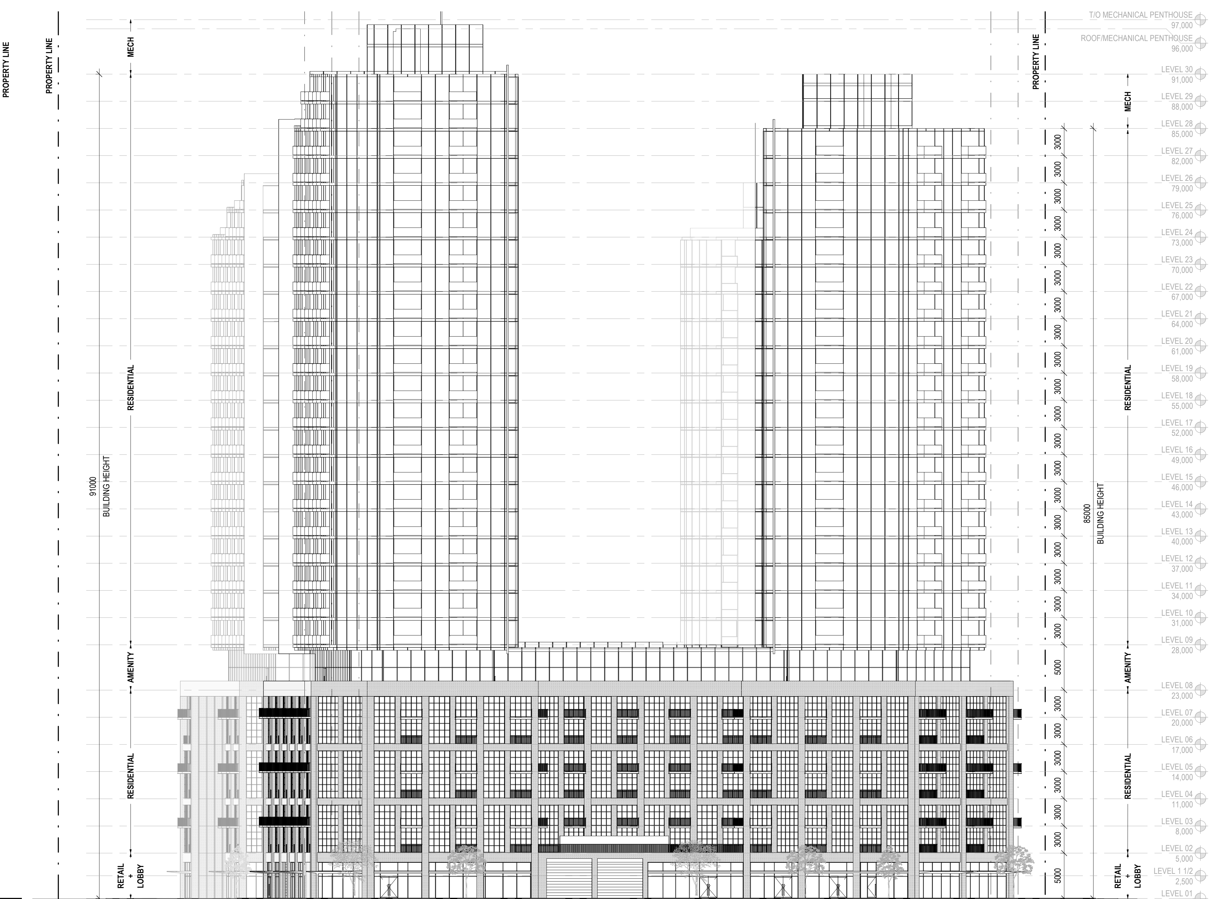
1 SITE ELEVATION - W SCALE: 1 : 250
