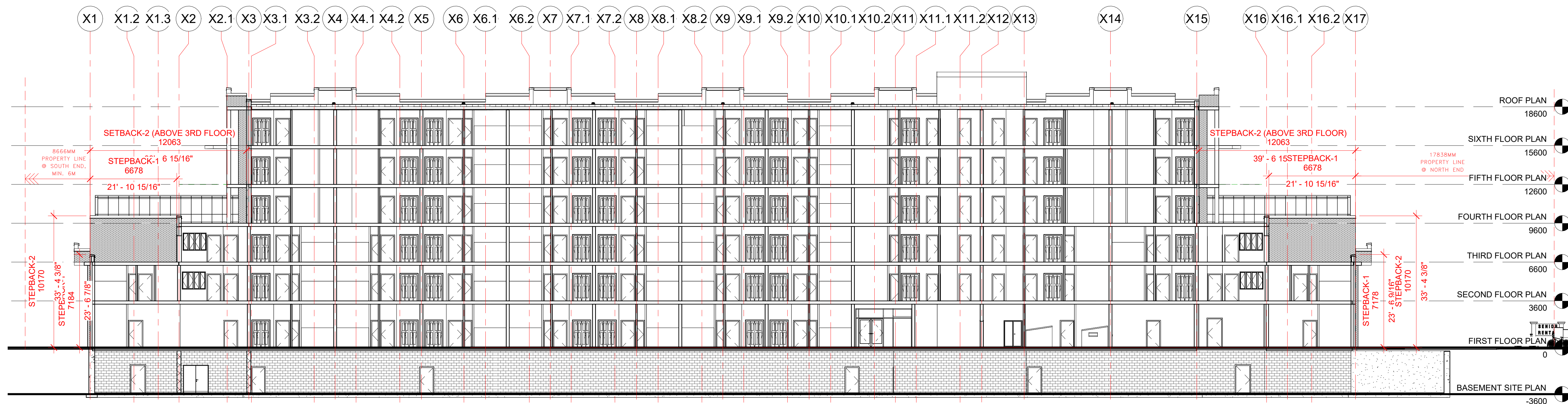
S4 Section 1 1 : 150
