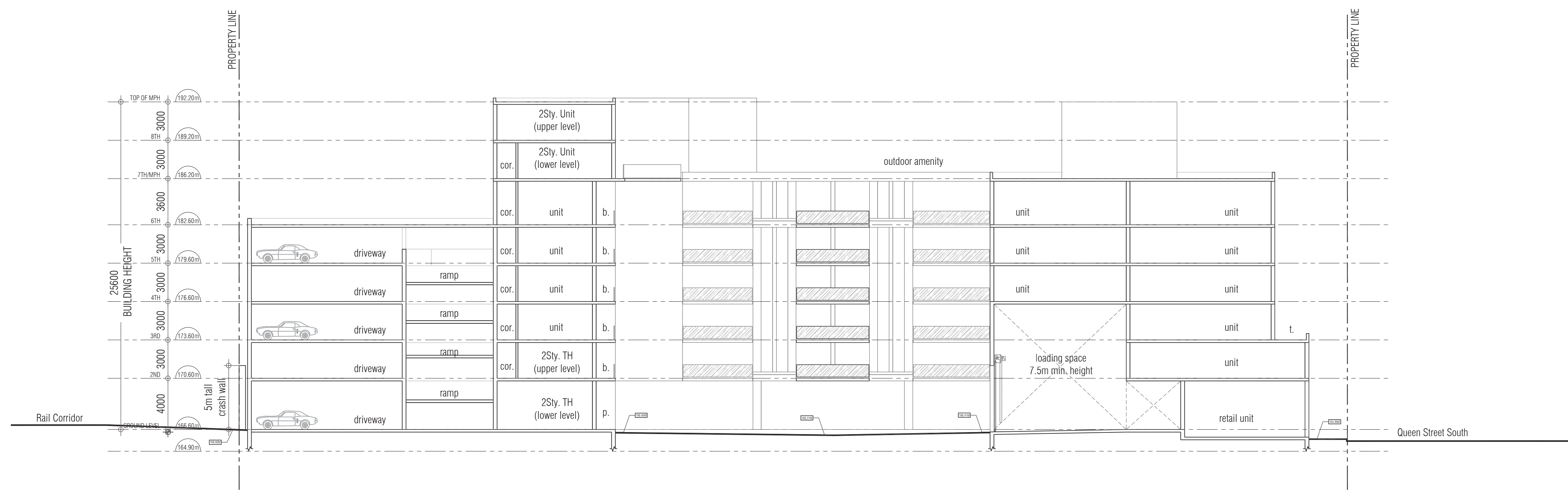
SECTION A-A 1 1:200 A501
