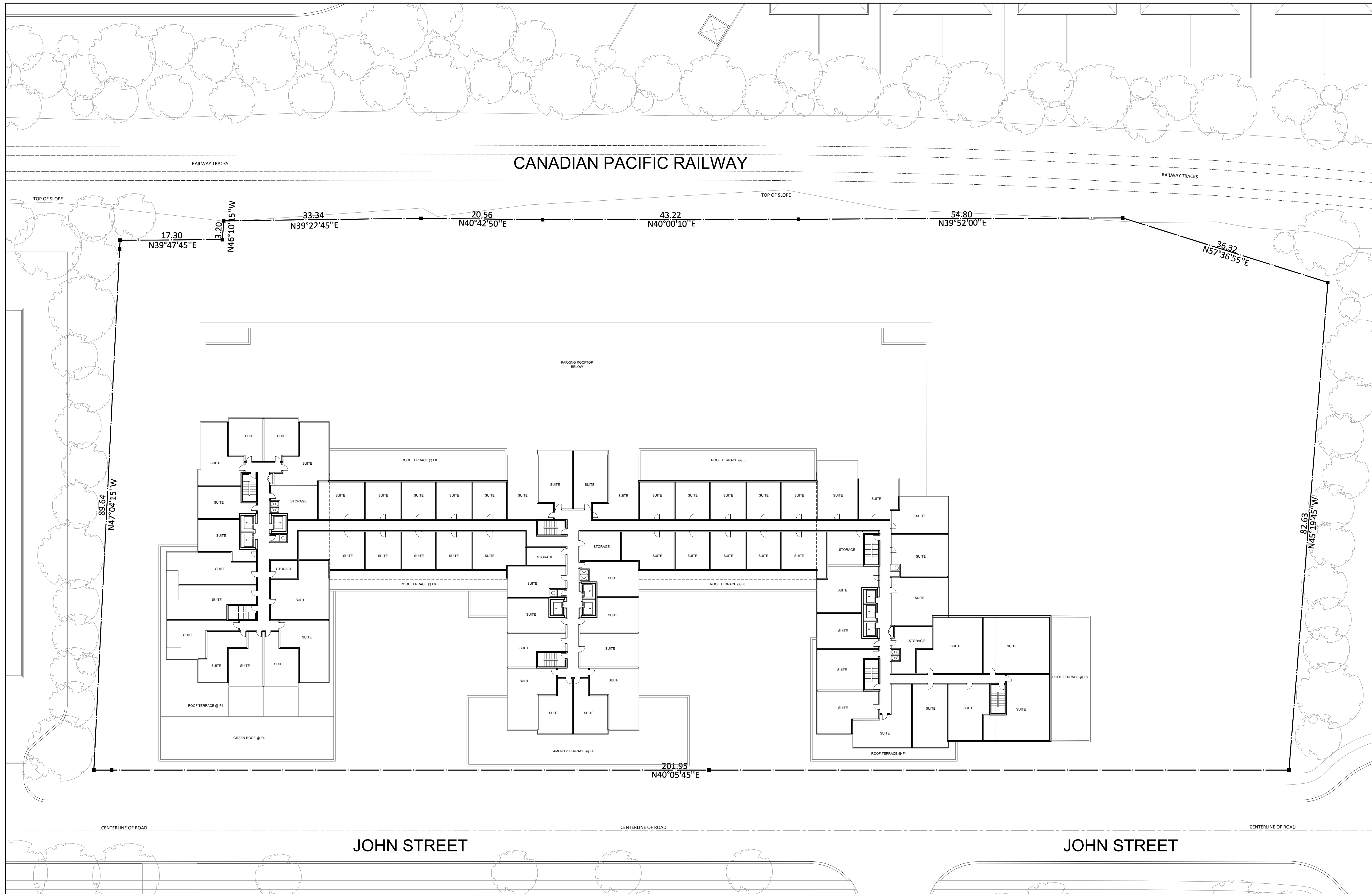
1 F10 FLOOR PLAN
