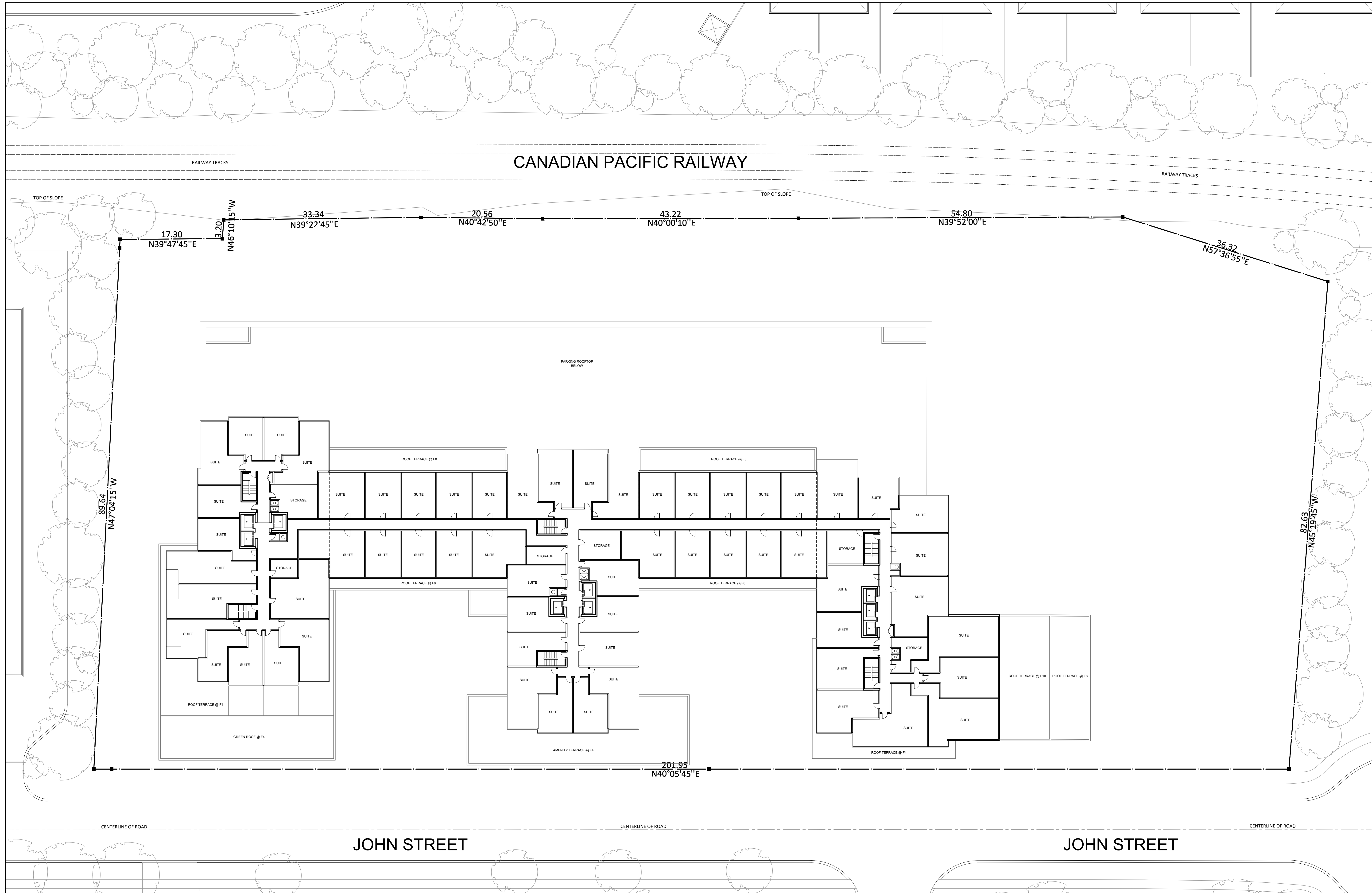
1 F11 FLOOR PLAN 1:300
