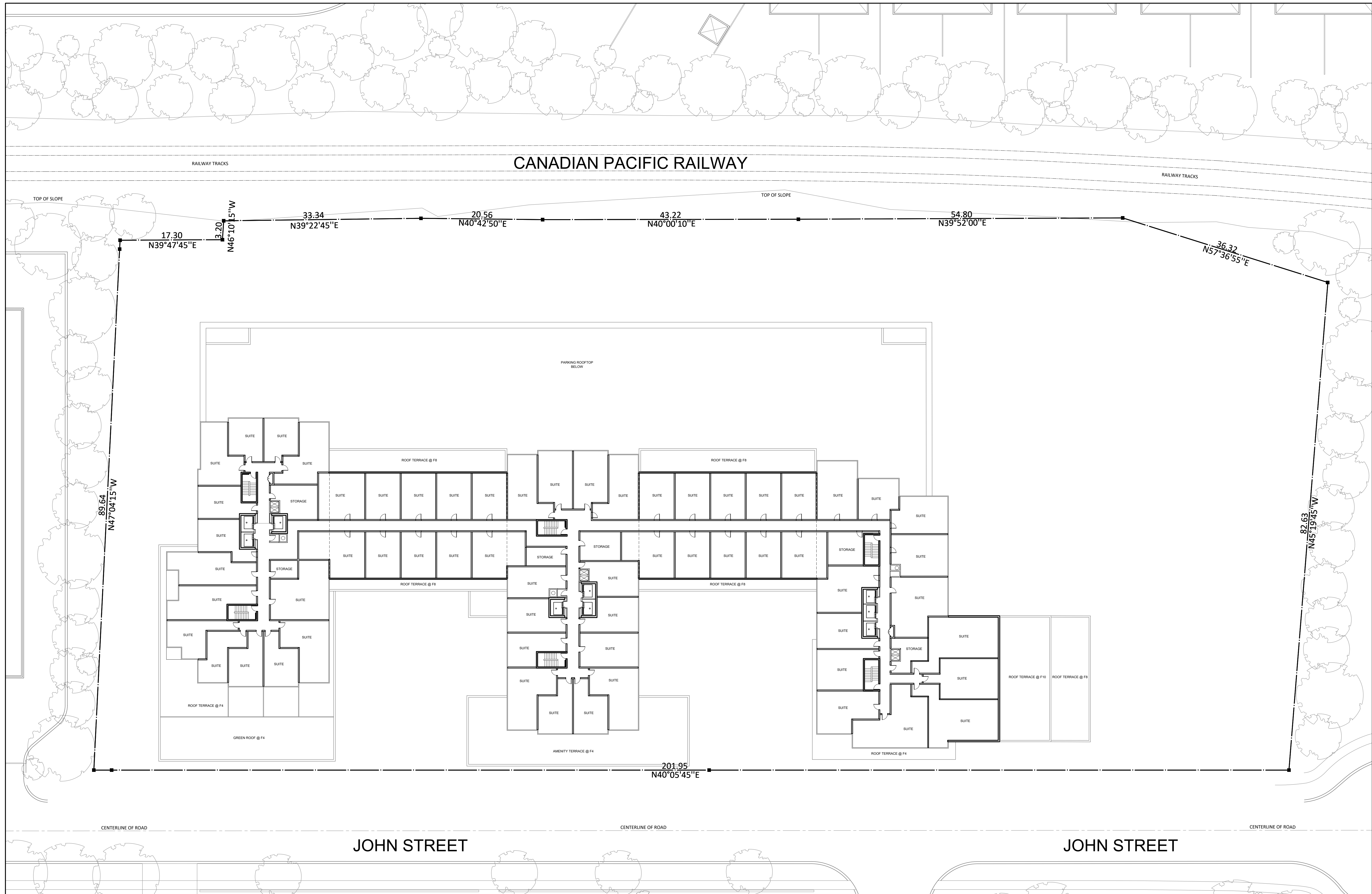
1 F12 FLOOR PLAN 1:300
