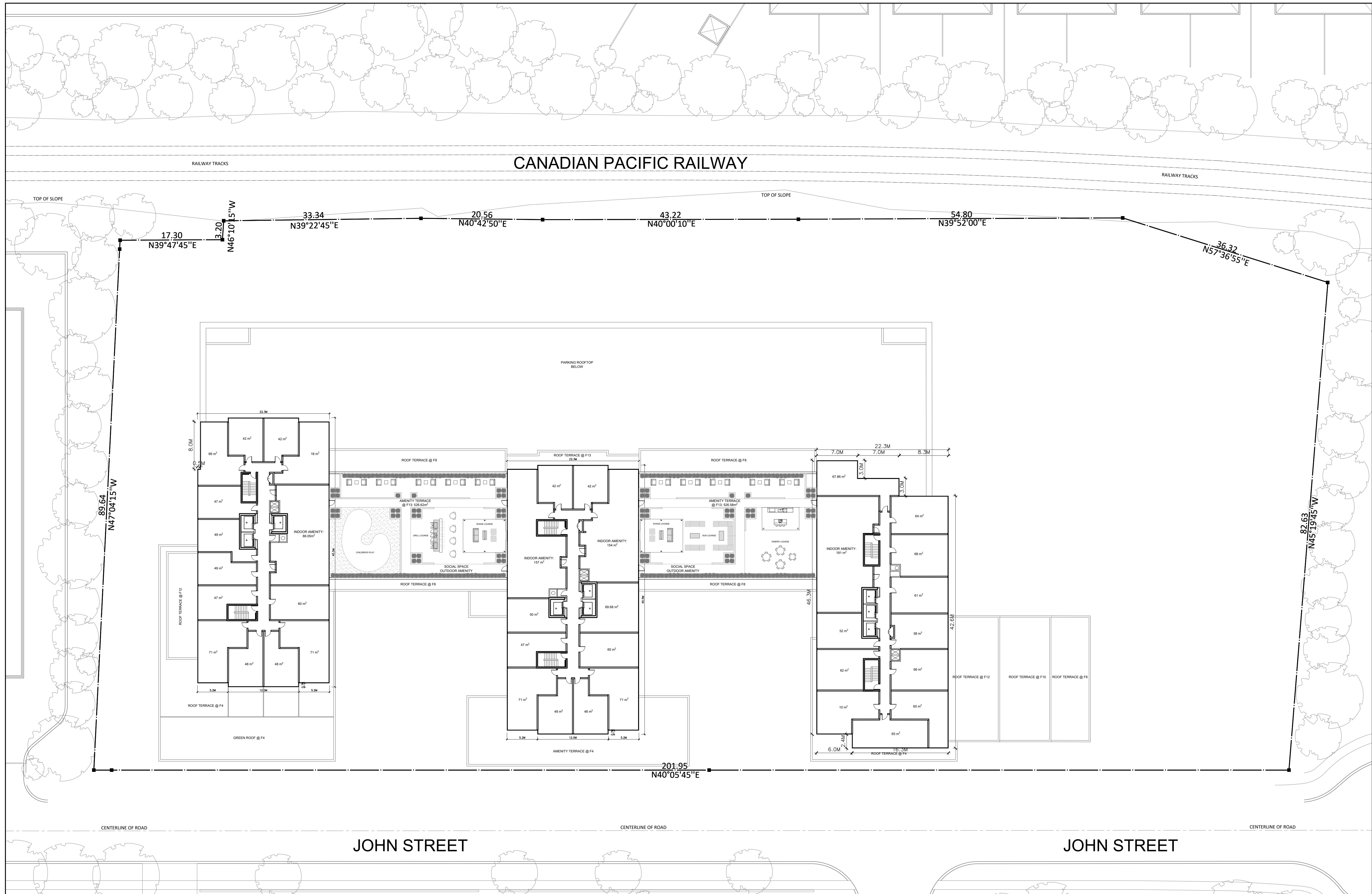
1 F13 ROOF TERRACE PLAN 1:300
