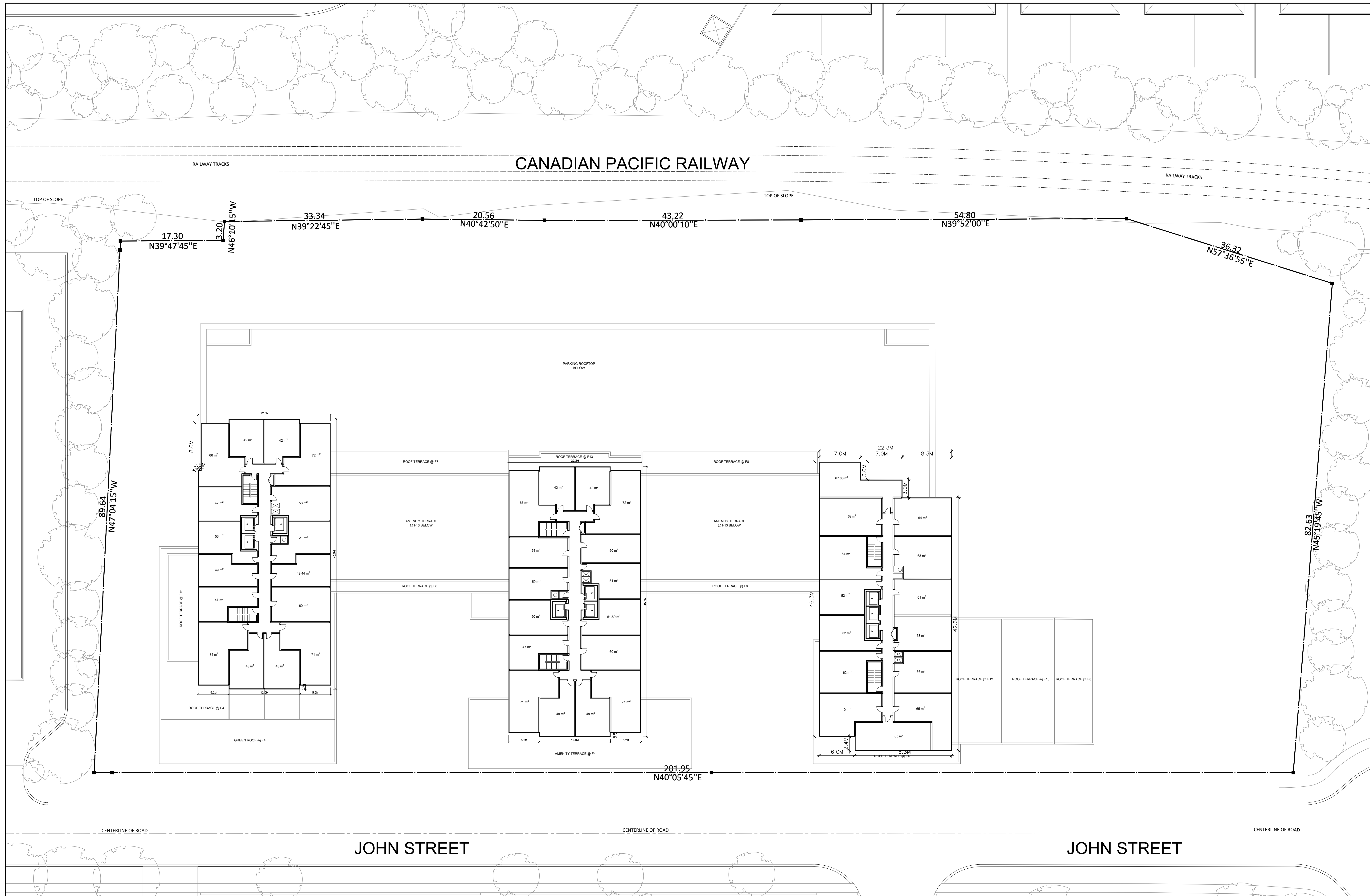
1 F14-F18 FLOOR PLAN 1:300
