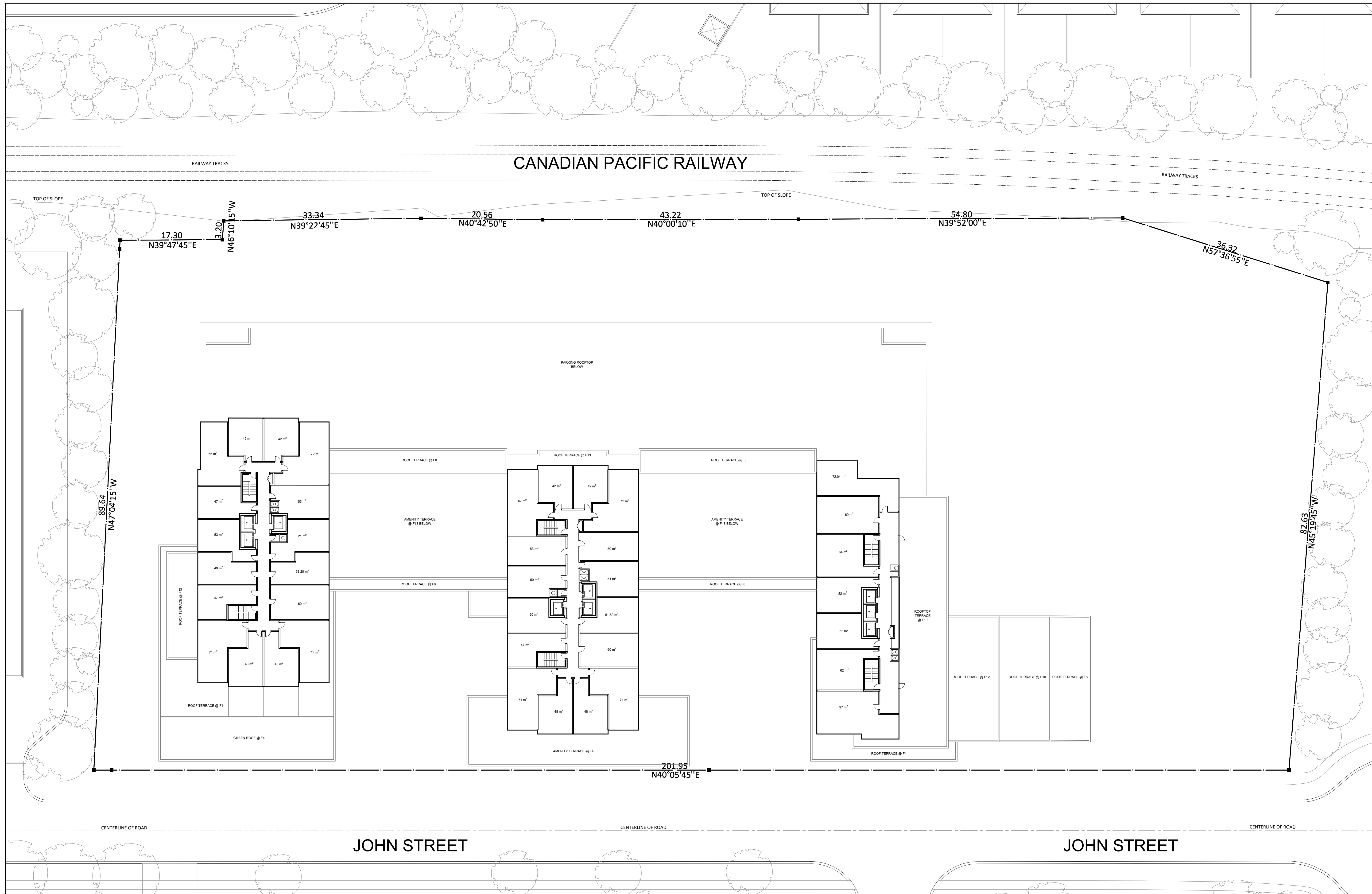
1 F19 FLOOR PLAN 1:300
