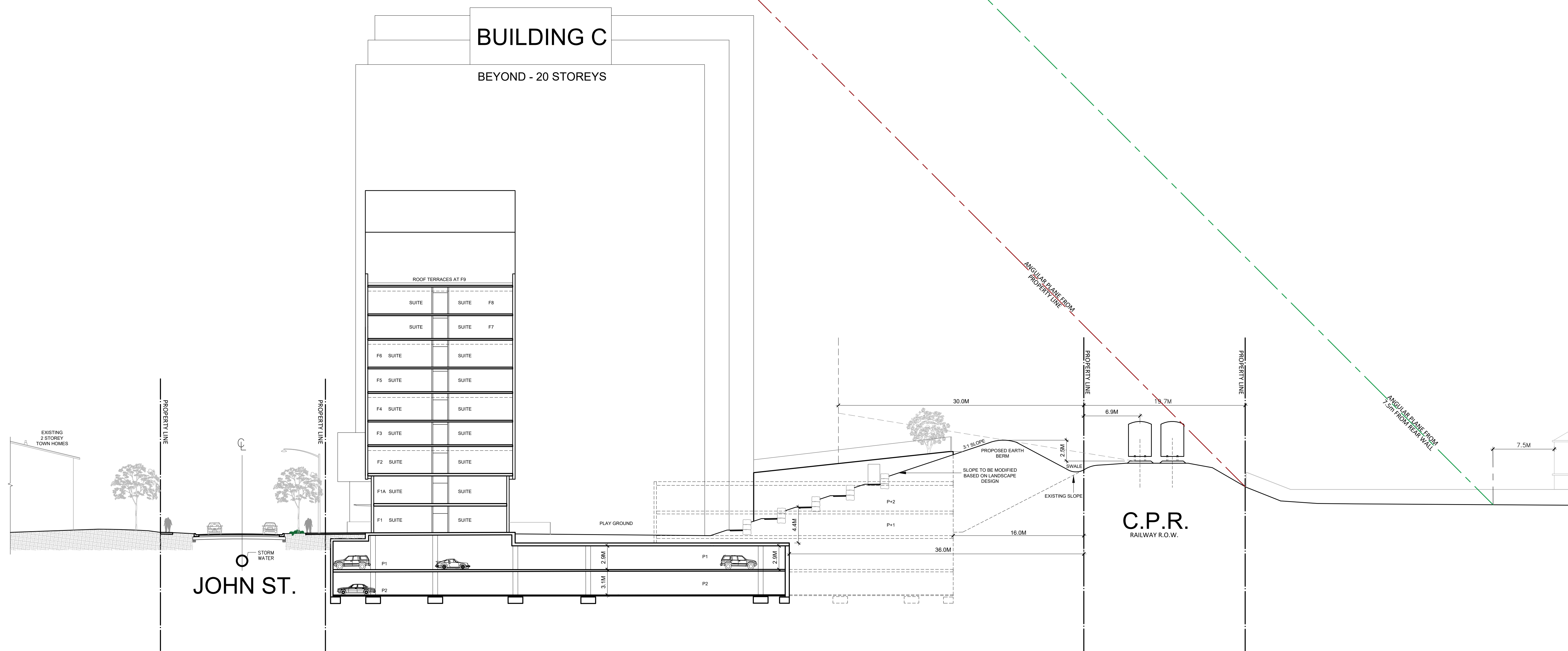
1 SECTION C-C Scale: 1:250
