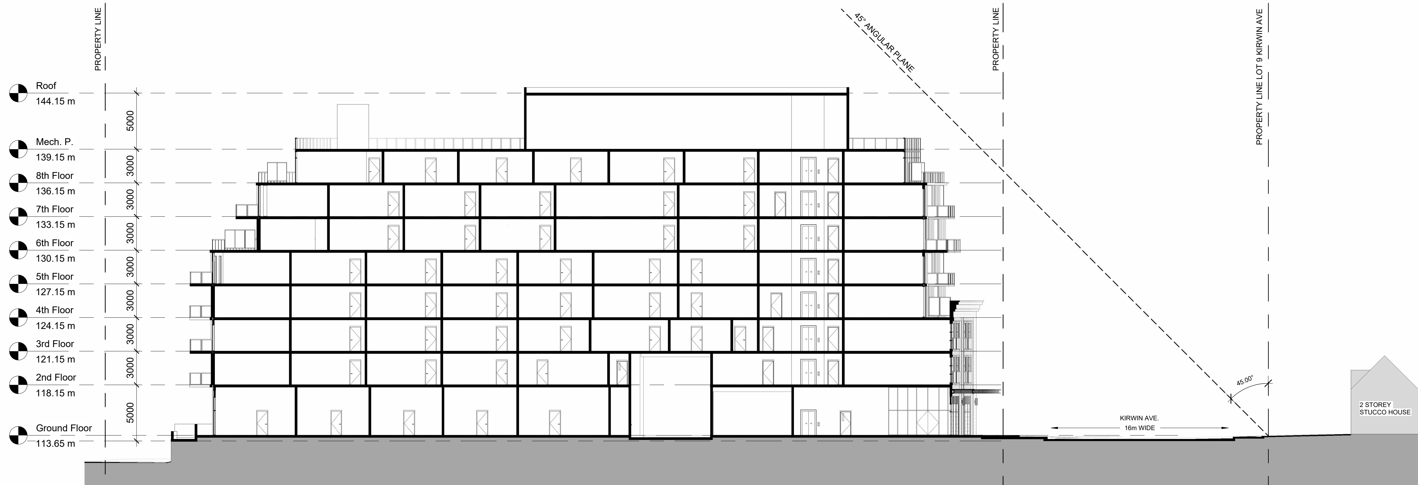
1 Site Section E/W 1 1 : 200
