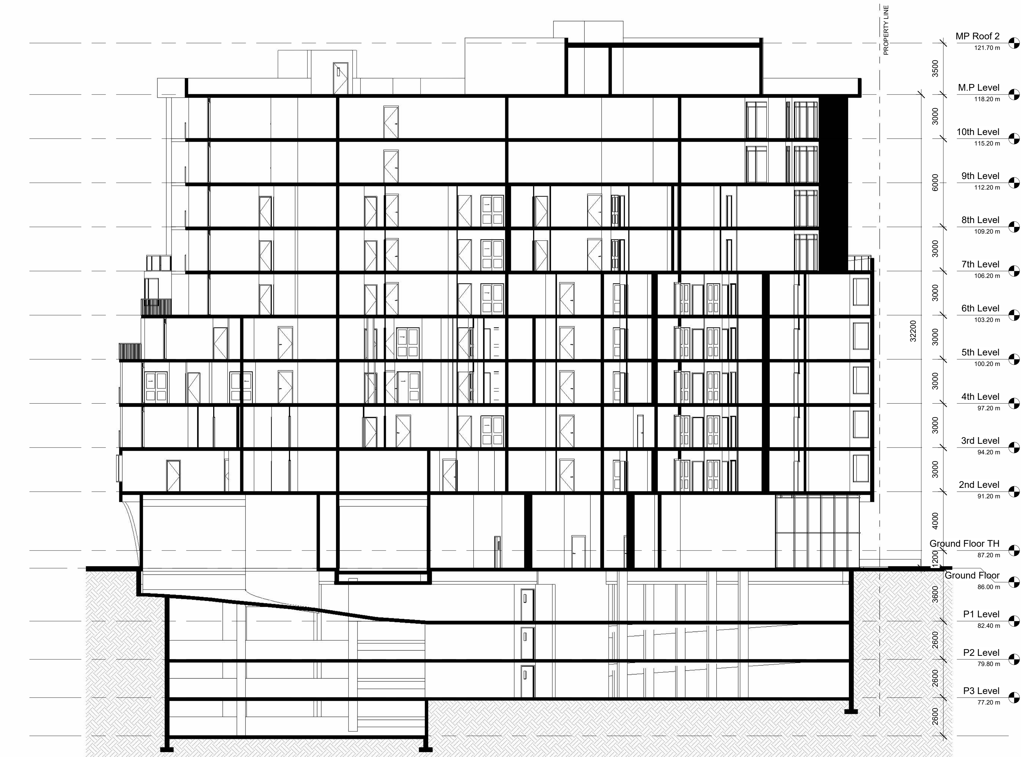
1 SECTION BB 1 : 150
