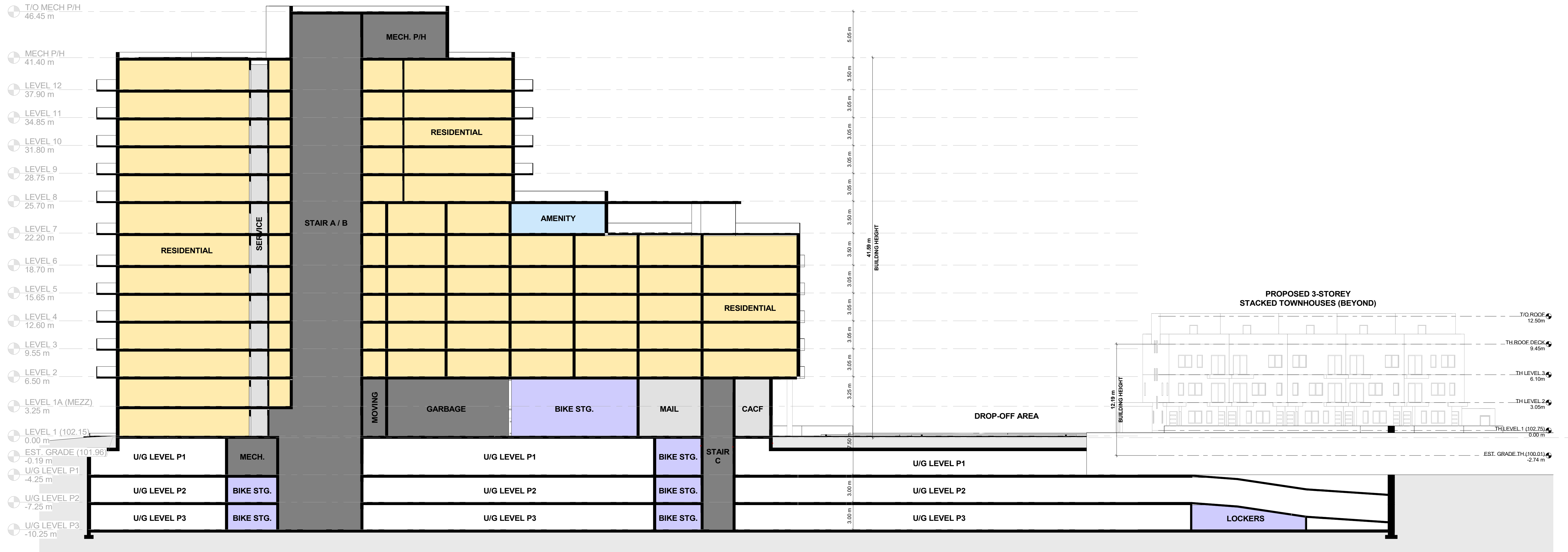
1 SITE SECTION 1 1 : 200
