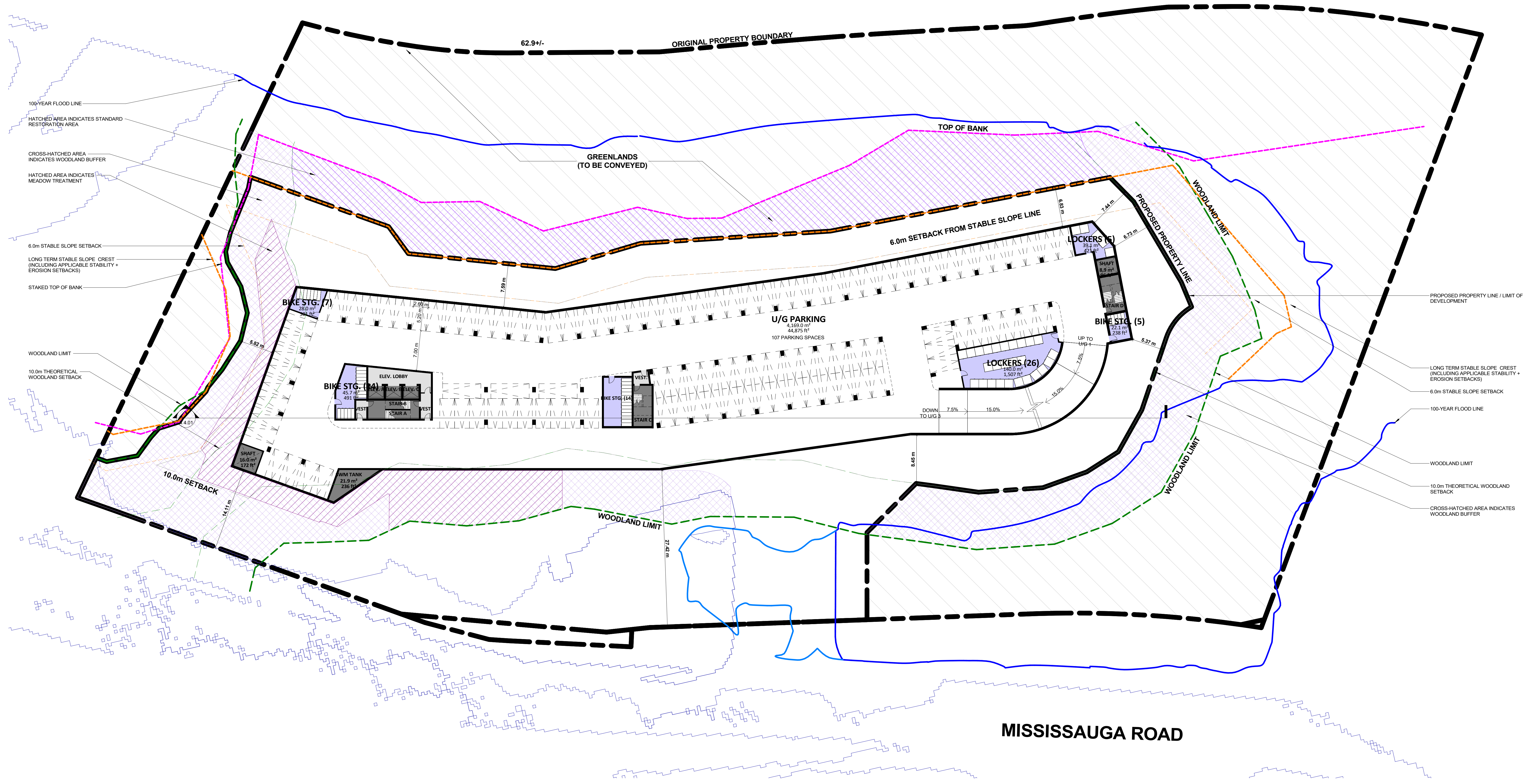
1 U/G LEVEL P2 1 : 300
