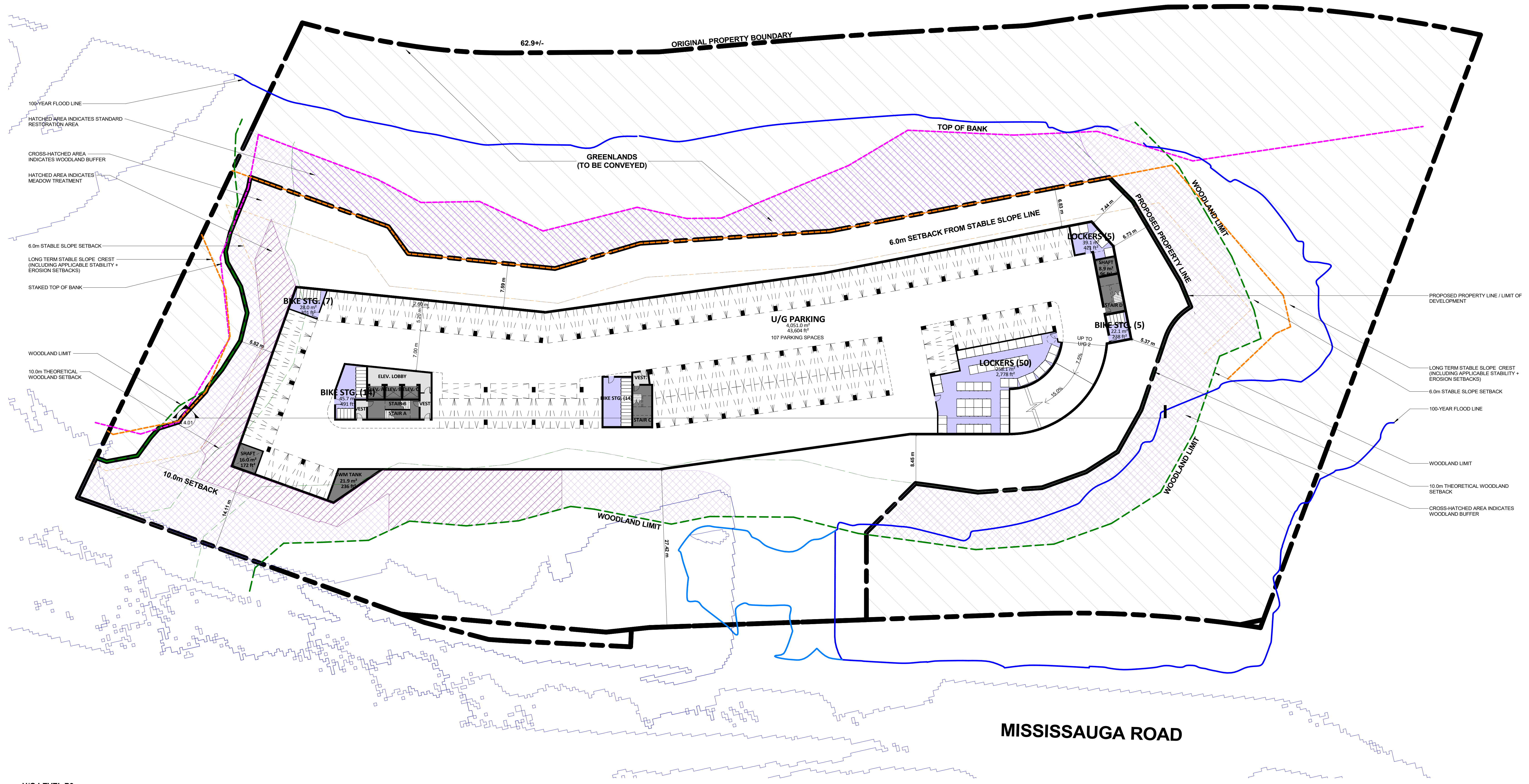
① U/G LEVEL P3 1 : 300
