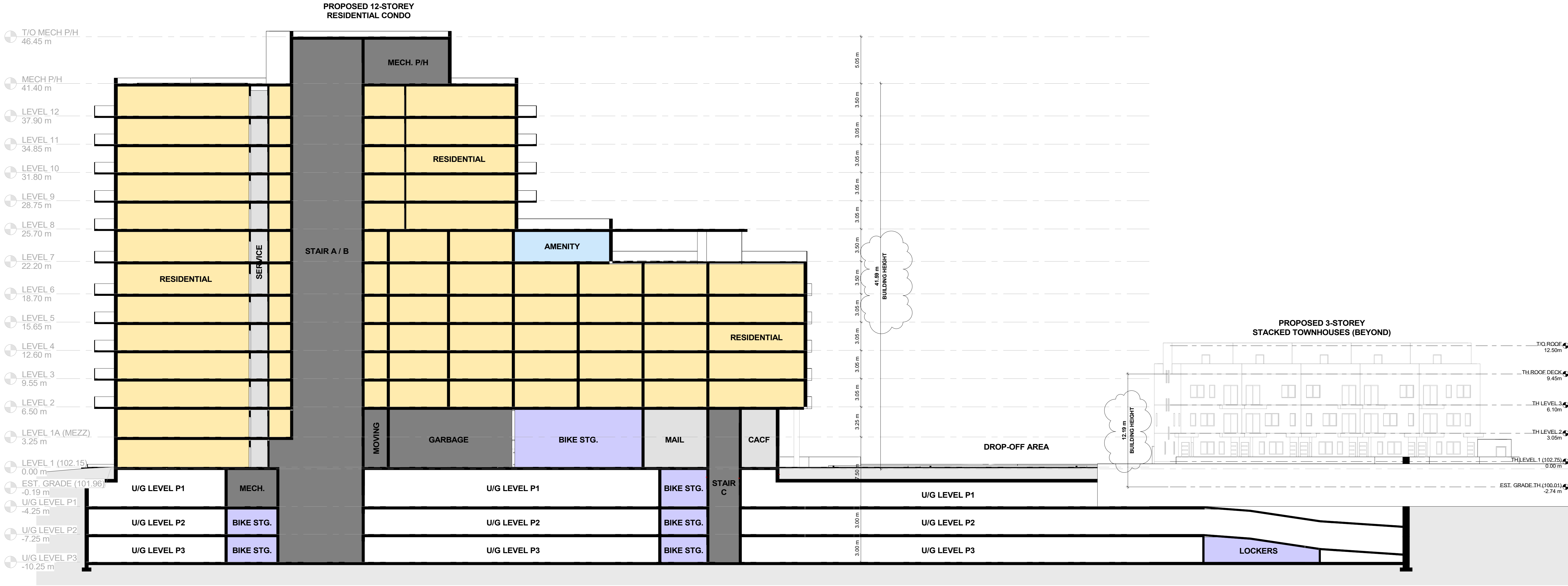
1 SITE SECTION 1 1 : 200
