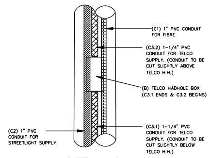
DETAIL 2 TELCO H.H.
