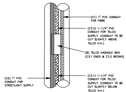
DETAIL 2 TELCO H.H.
