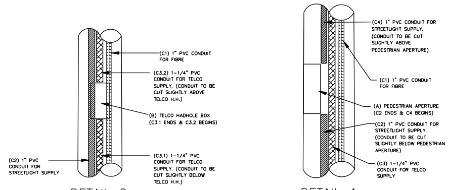
DETAIL 2 TELCO H.H.
