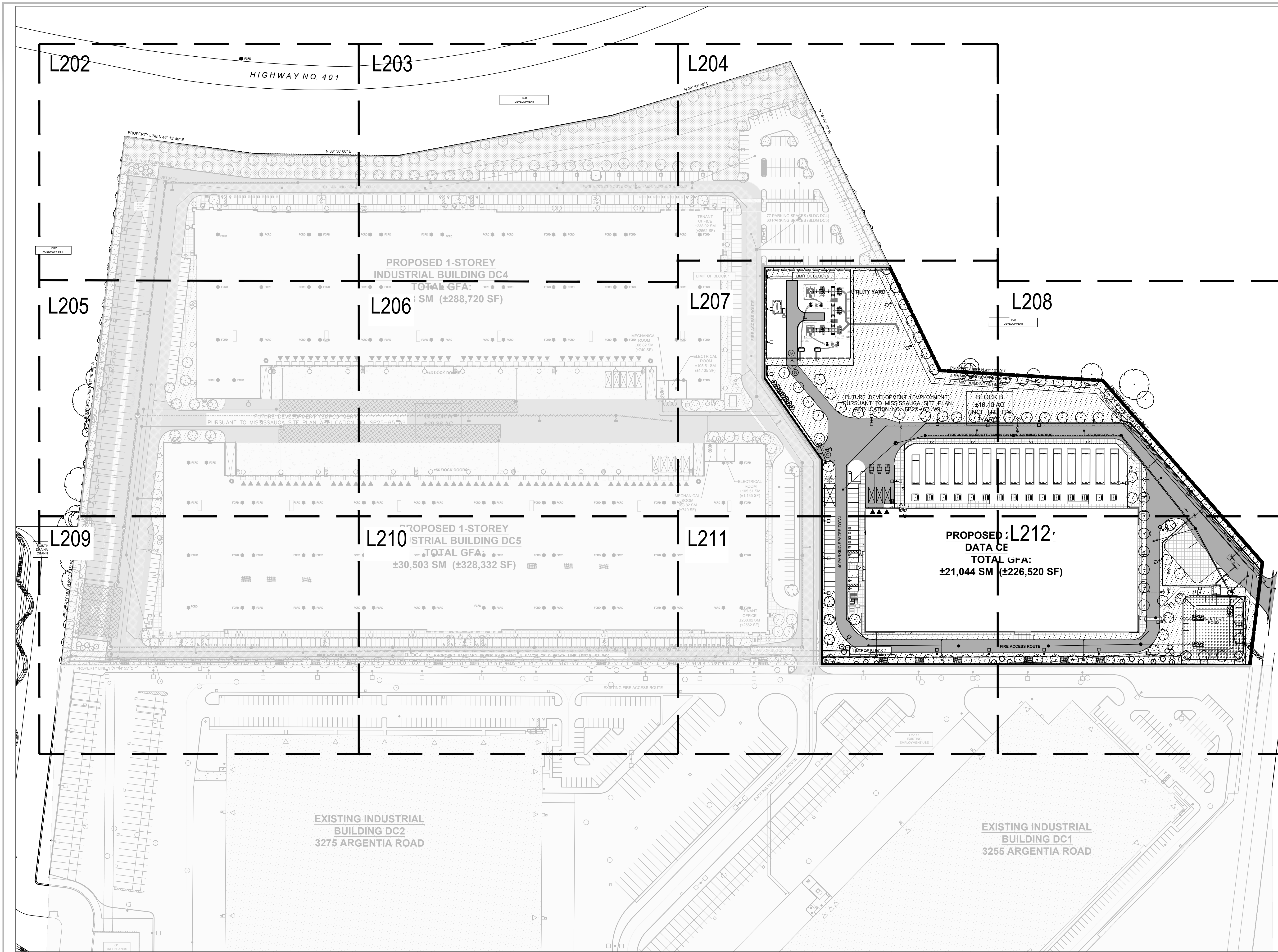
1 LANDSCAPE PLAN L-201 1:1500
