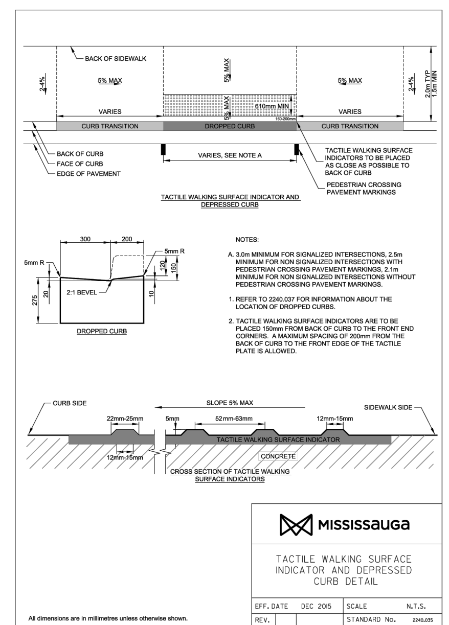
4 TACTILE WALKING SURFACE N.T.S.
