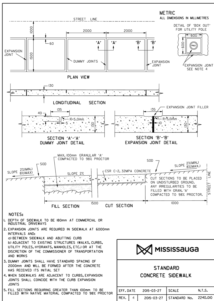
1 STANDARD CONCRETE SIDEWALK N.T.S.
