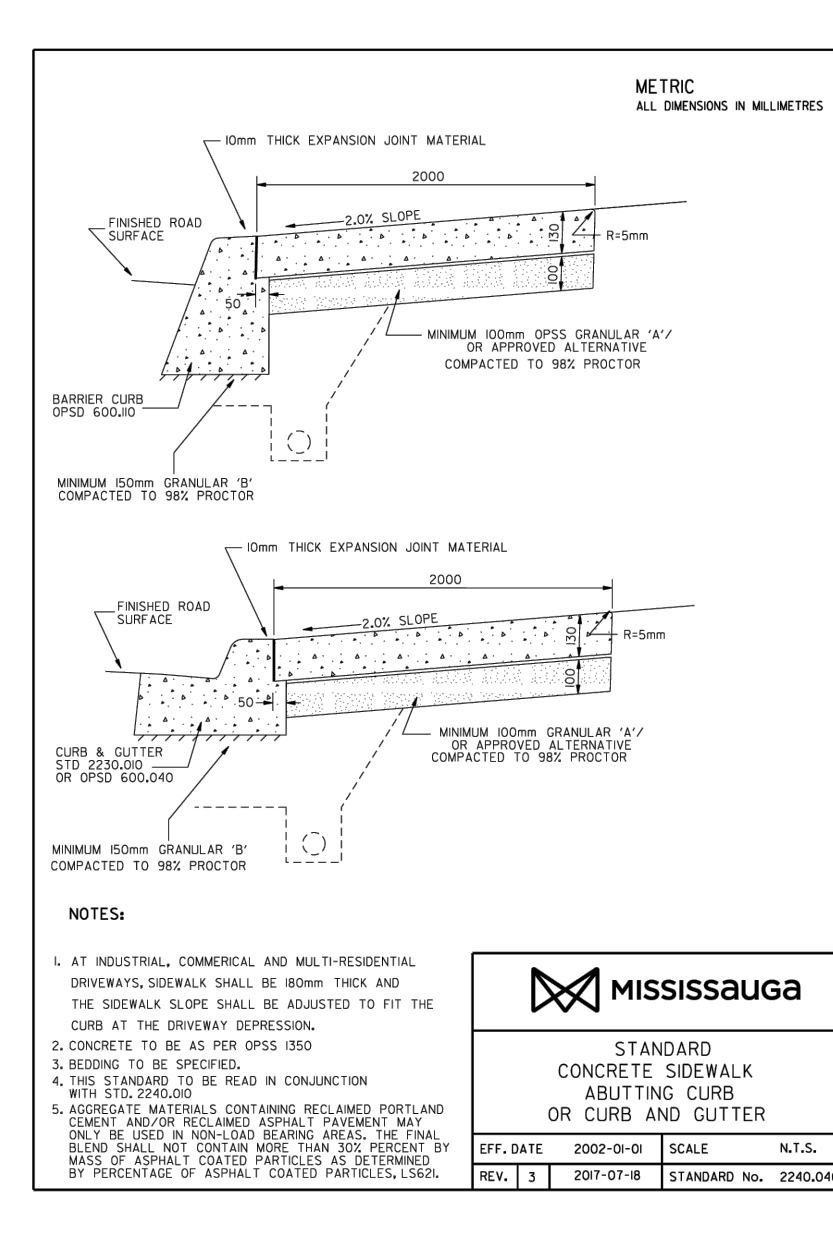
2 STANDARD CONCRETE CURB N.T.S.
