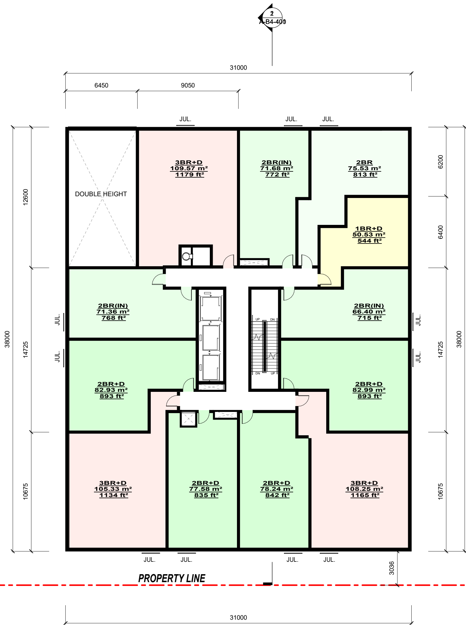
2 LEVEL 3 1 : 200
